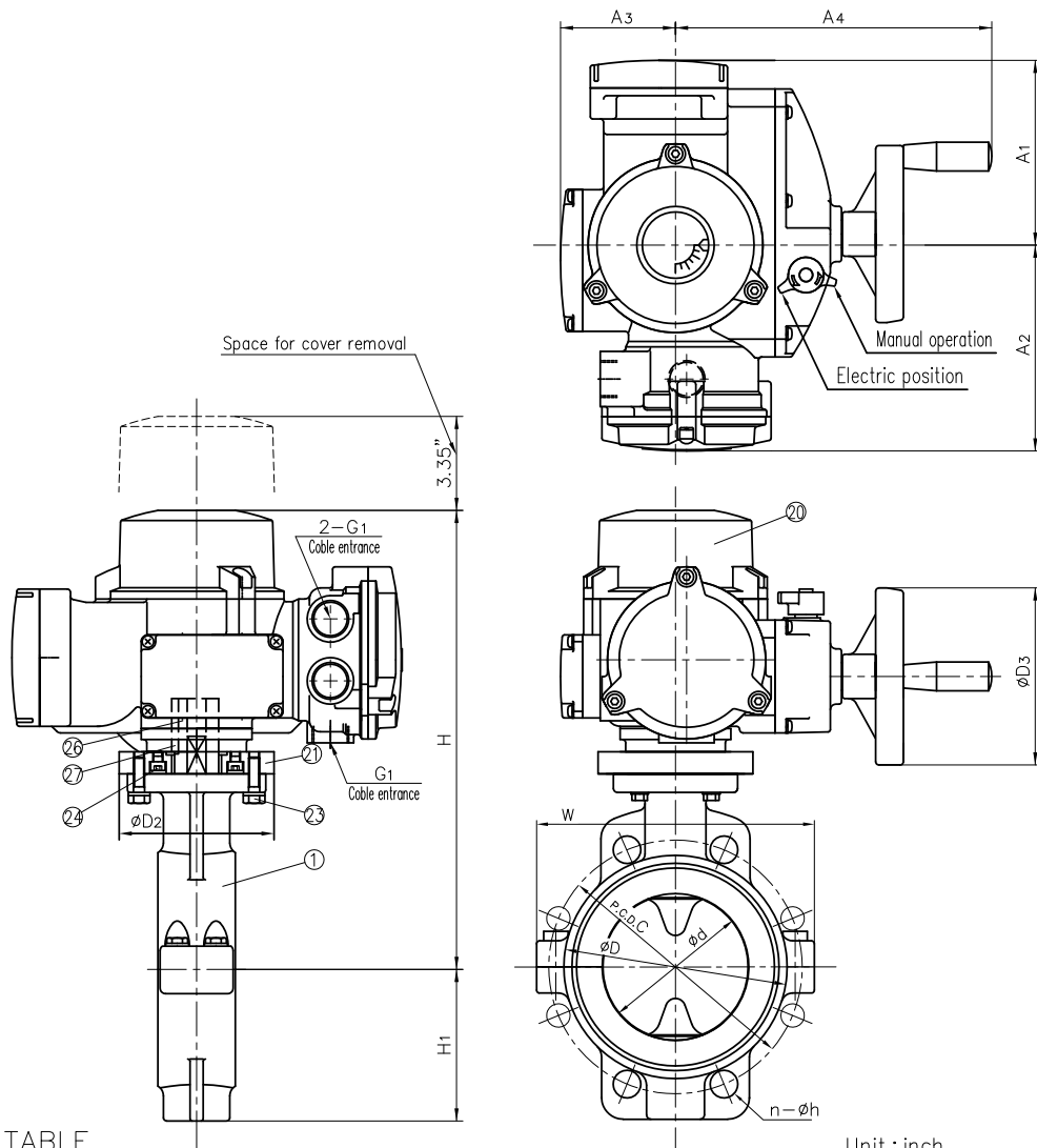
DIMENSIONS TABLE
